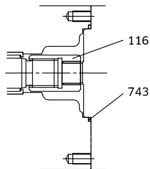
SAE 'A' T/D KIT
